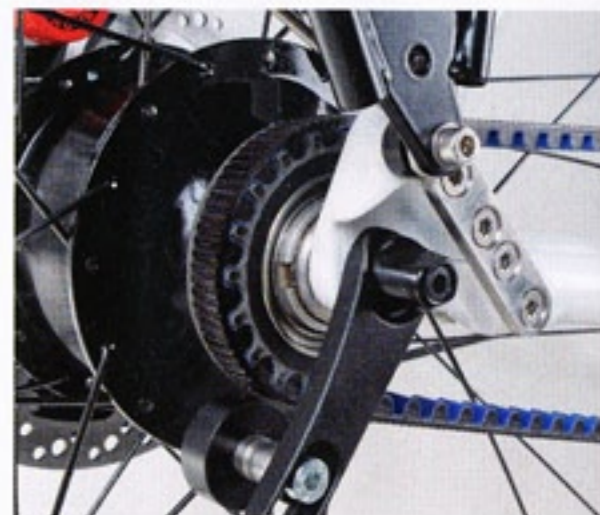
Rahmenkupplung für den Riementausch. Der Snubber verhindert ein Überspringen.
